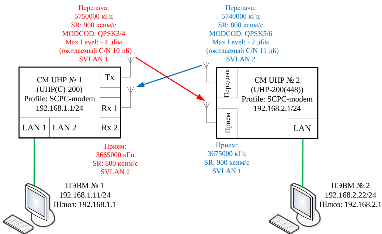
Рисунок 3. Сеть топологии «точка-точка», построенная на CM UHP-200 в составе ЗССС С-диапазона
